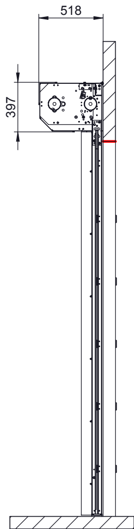
SECTION A-A
