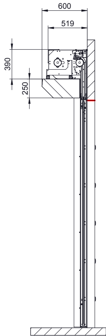
SECTION A-A
